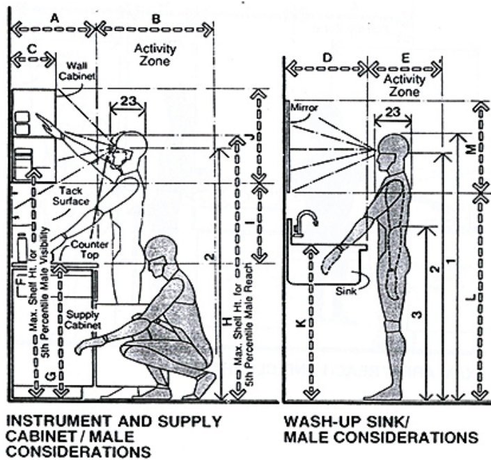
รูปที่ 8.2.3 ขนาดและระยะต่างๆ ของร่างกายมนุษย์ที่สัมพันธ์กับ ครุภัณฑ์ เครื่องมือและอุปกรณ์ต่างๆ ในห้องปฏิบัติการ สำหรับเพศชาย (ที่มา Human dimension & interior space, 1979: หน้า 236)
