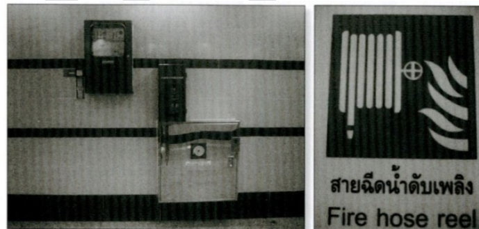
รูปที่ 10.27 การติดตั้งตู้สายฉีดน้ำดับเพลิง
